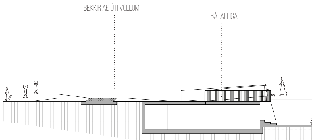
SNEIDING A-A Í RAMP
