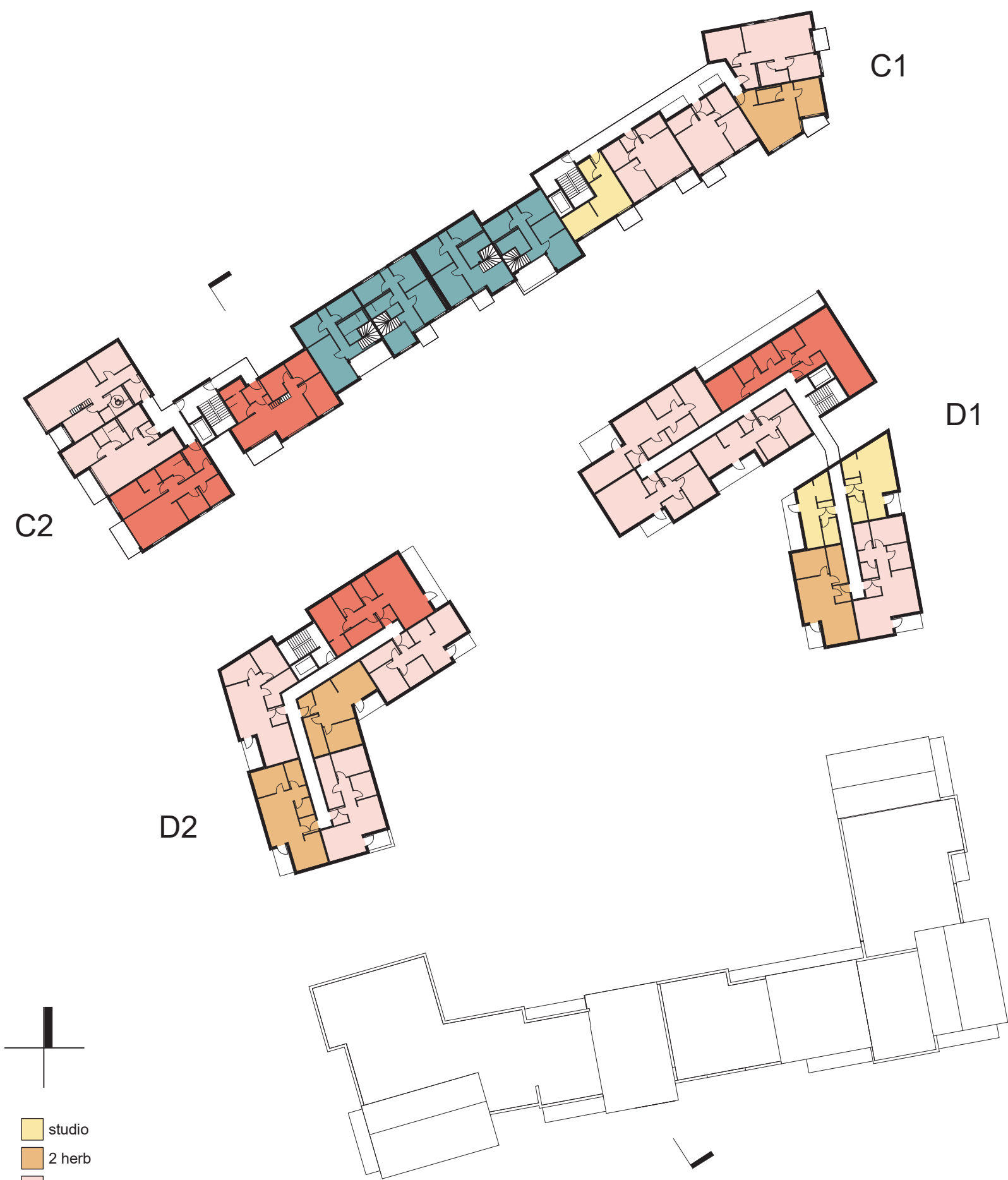
GRUNNMYND 4. HÆÐ D-REITUR / 3. HÆÐ C-REITUR MKV. 1:500
