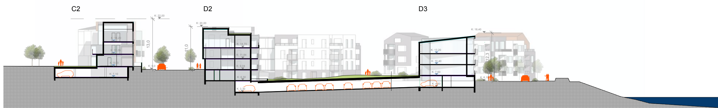
SNIÐ MKV. 1:500
