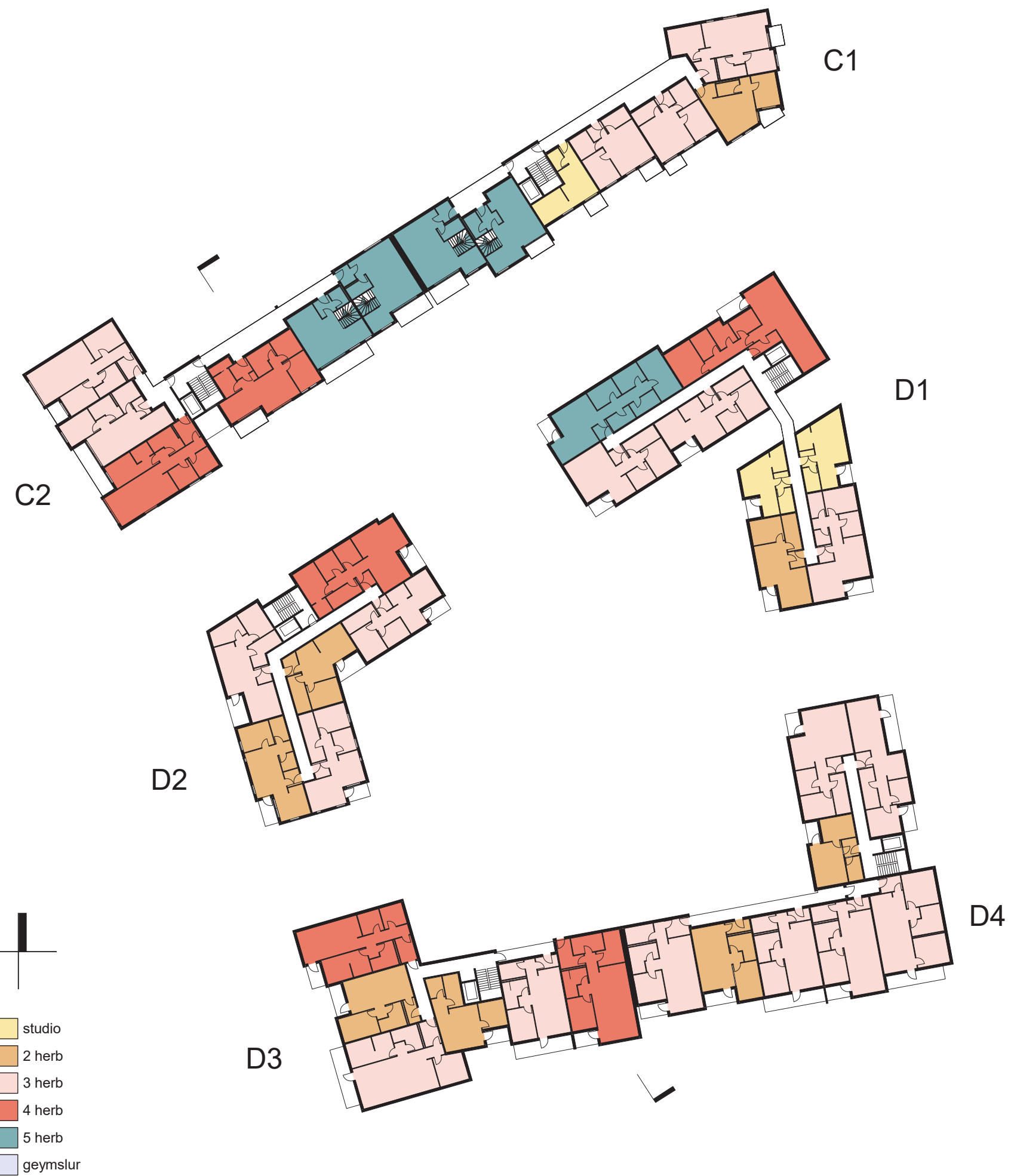
GRUNNMYND 3. HÆÐ D-REITUR / 2. HÆÐ C-REITUR MKV. 1:500
