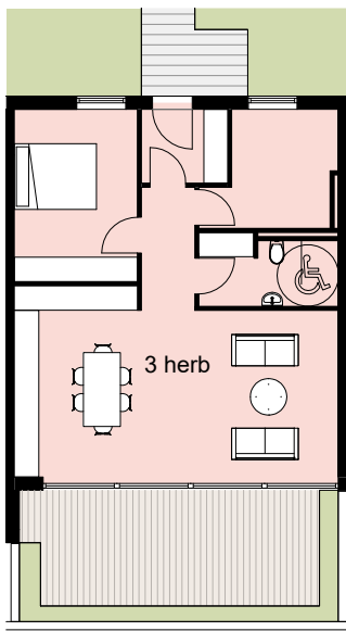
C-REITUR JARÐHÆÐ
