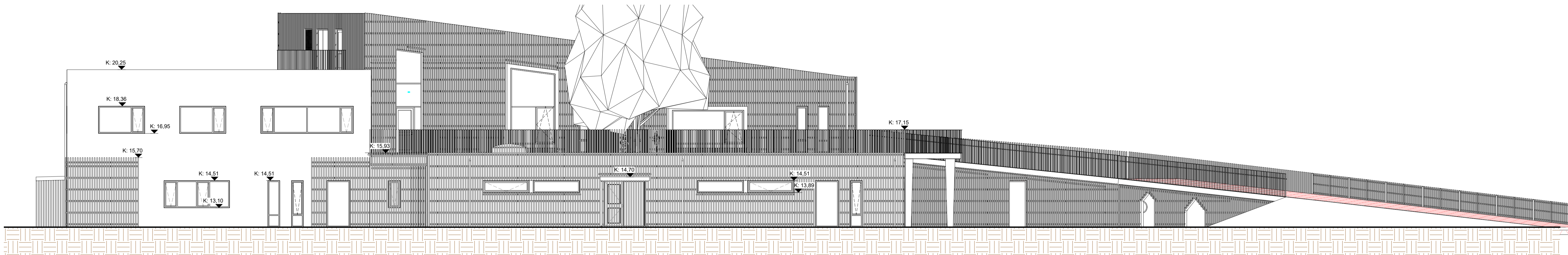
SUDUR - VESTUR 1 : 100
